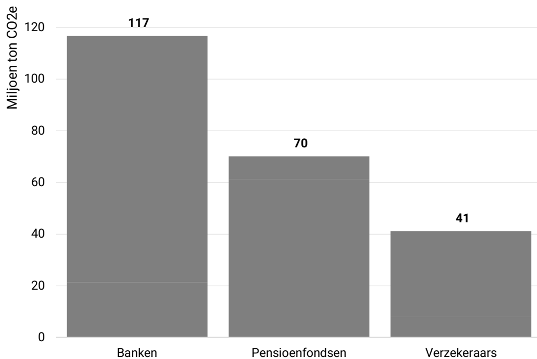
Figuur 1: Gefinancierde uitstoot (scope 1 en 2) van de Nederlandse financiële sector per type financier
